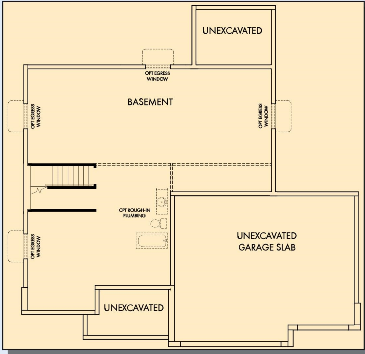
OPTIONAL BASEMENT
