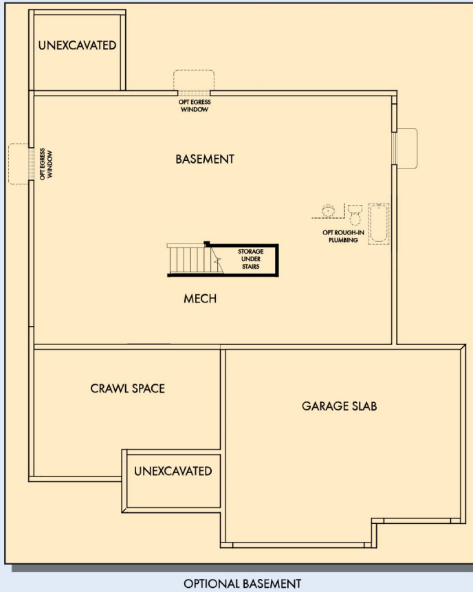
OPTIONAL BASEMENT
